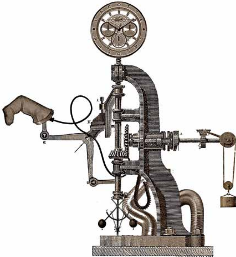
Fig. 12. MACHINE A TATER DIT "TATEUSE"
